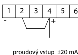
Obr. 2. Různé způsoby připojení vstupů přístroje.
